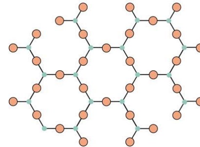
crystalline SiO 2
