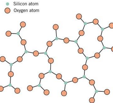
noncrystalline SiO 2
